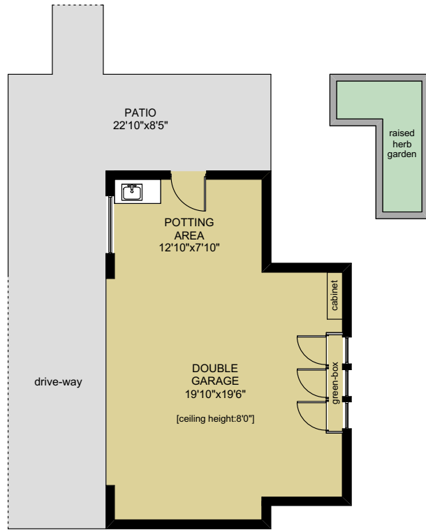
GARAGE 594 SQ.FT
